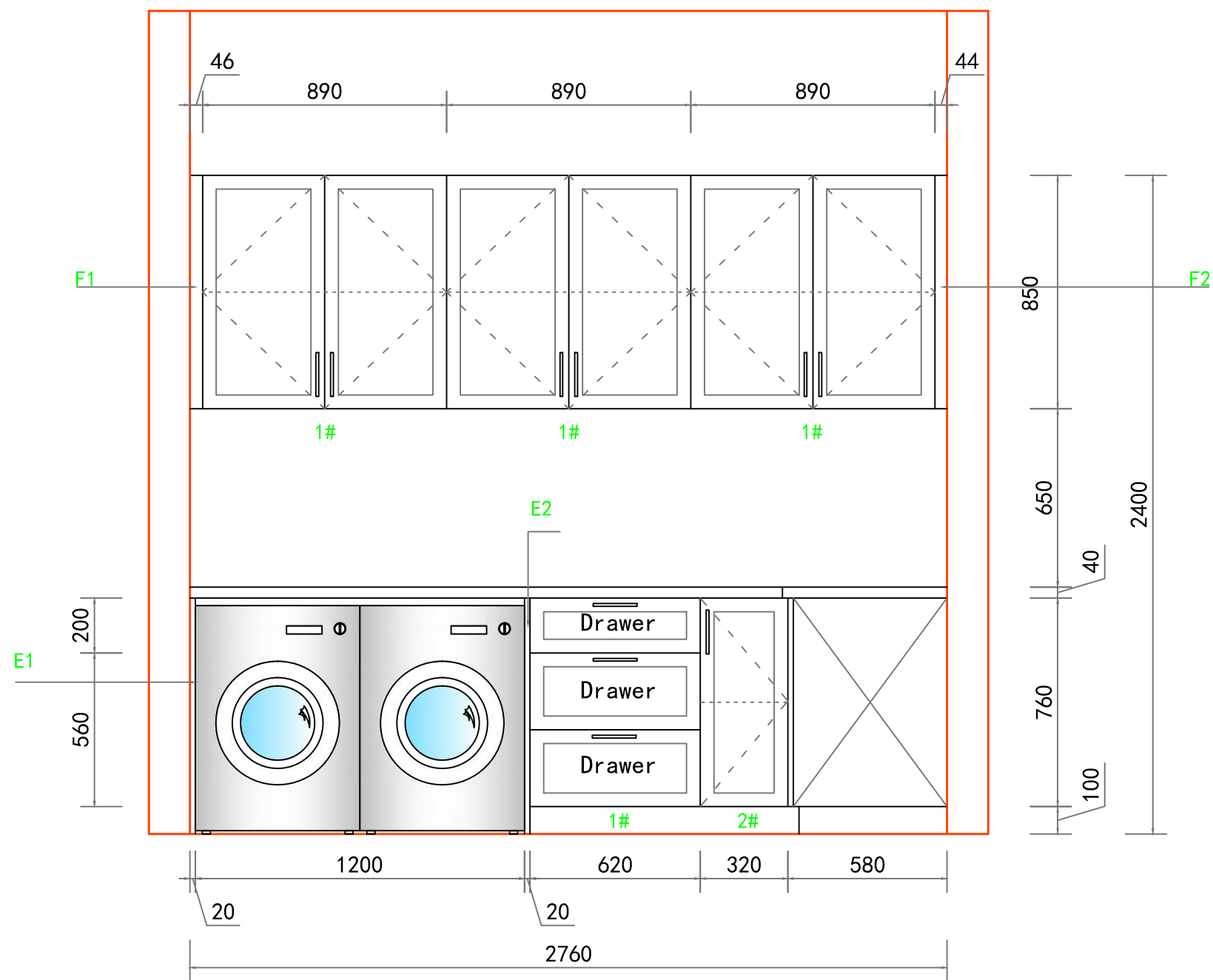
ELEVATION A
