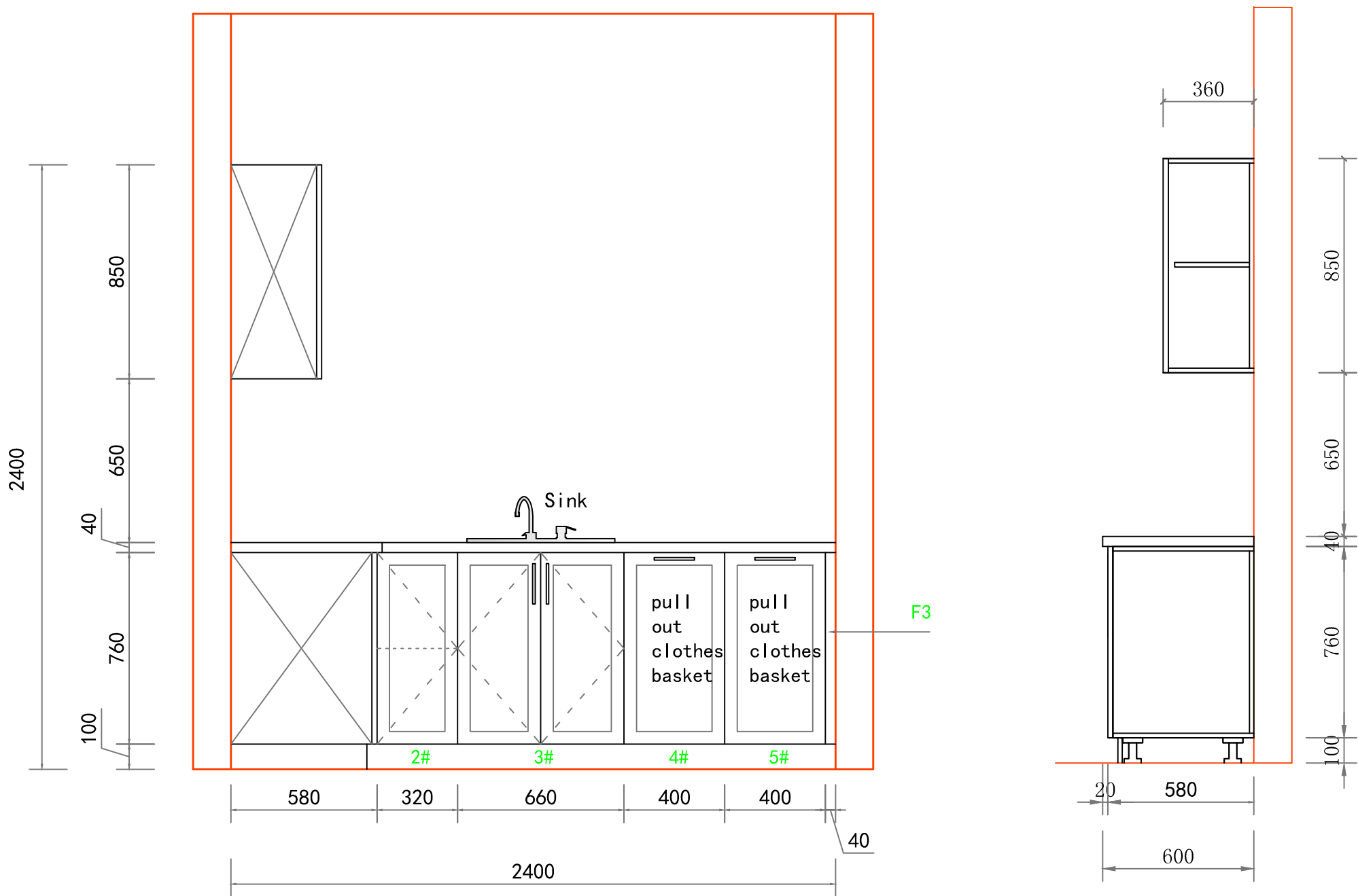
ELEVATION B
